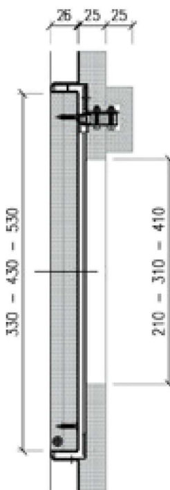
SEZIONE VERTICALE
