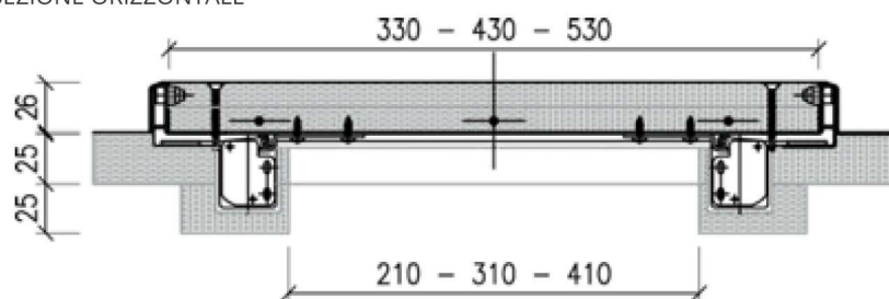
SEZIONE ORIZZONTALE
